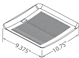
Fan Grille
